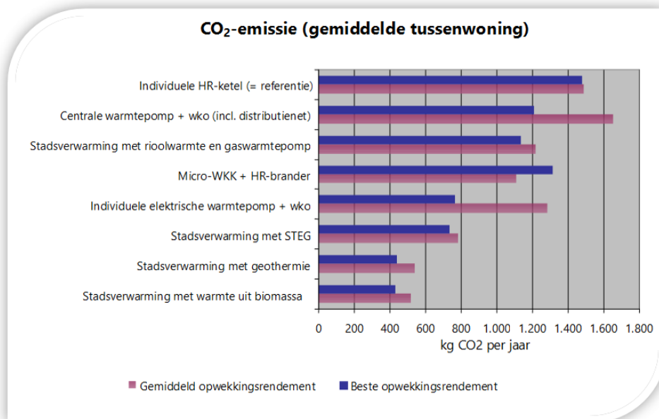
Figuur 2 : Verschillende mogelijkheden voor het verwarmen van een woning
